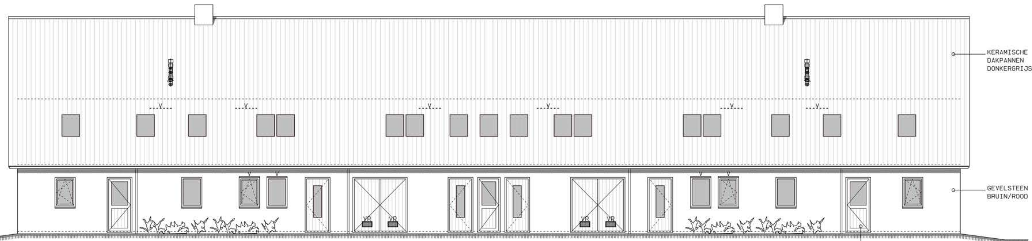
NOORDGEVEL
