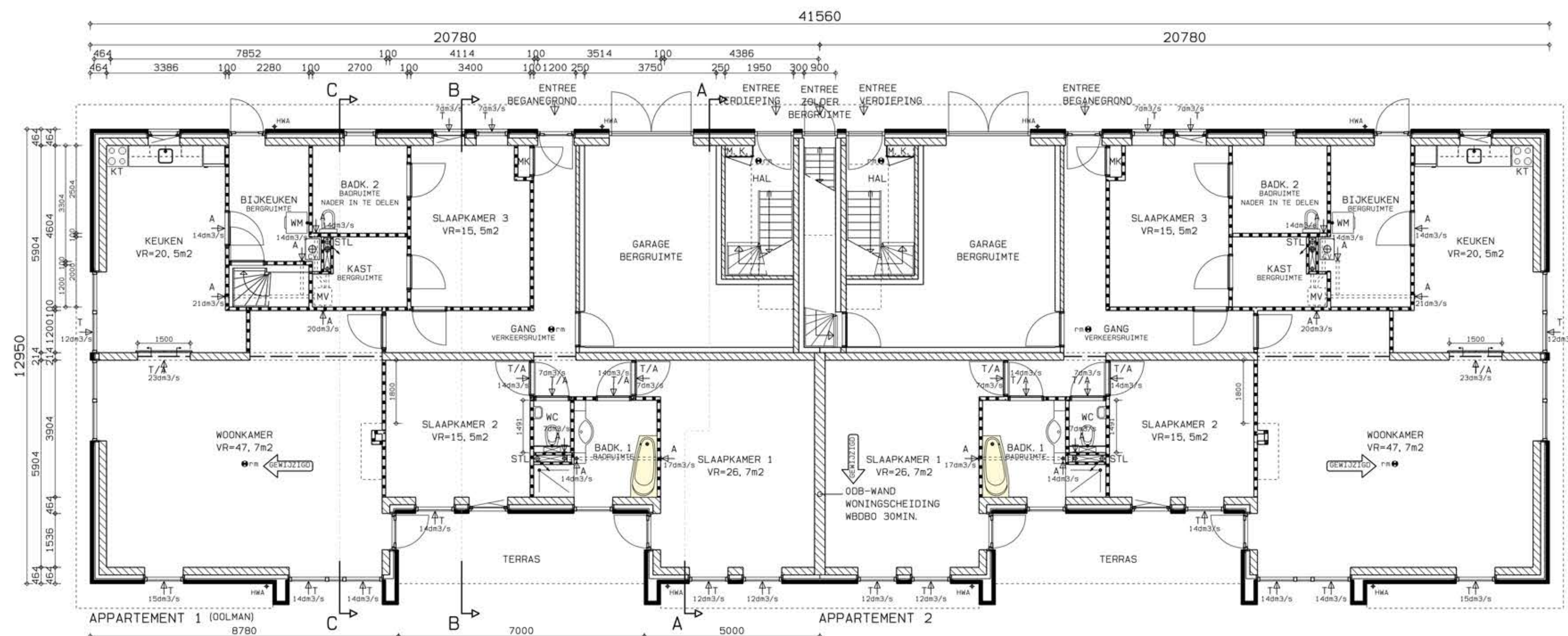
BEGANEGROND
