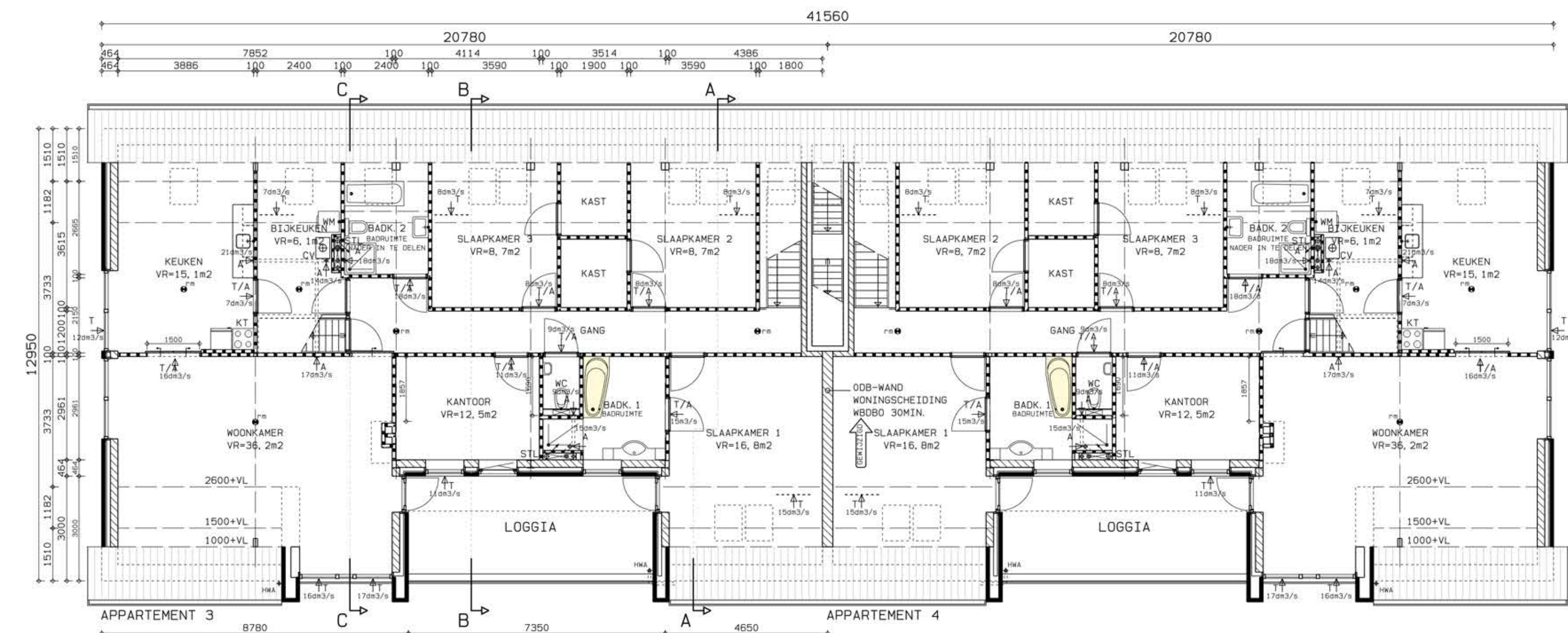
VERDIEPING
